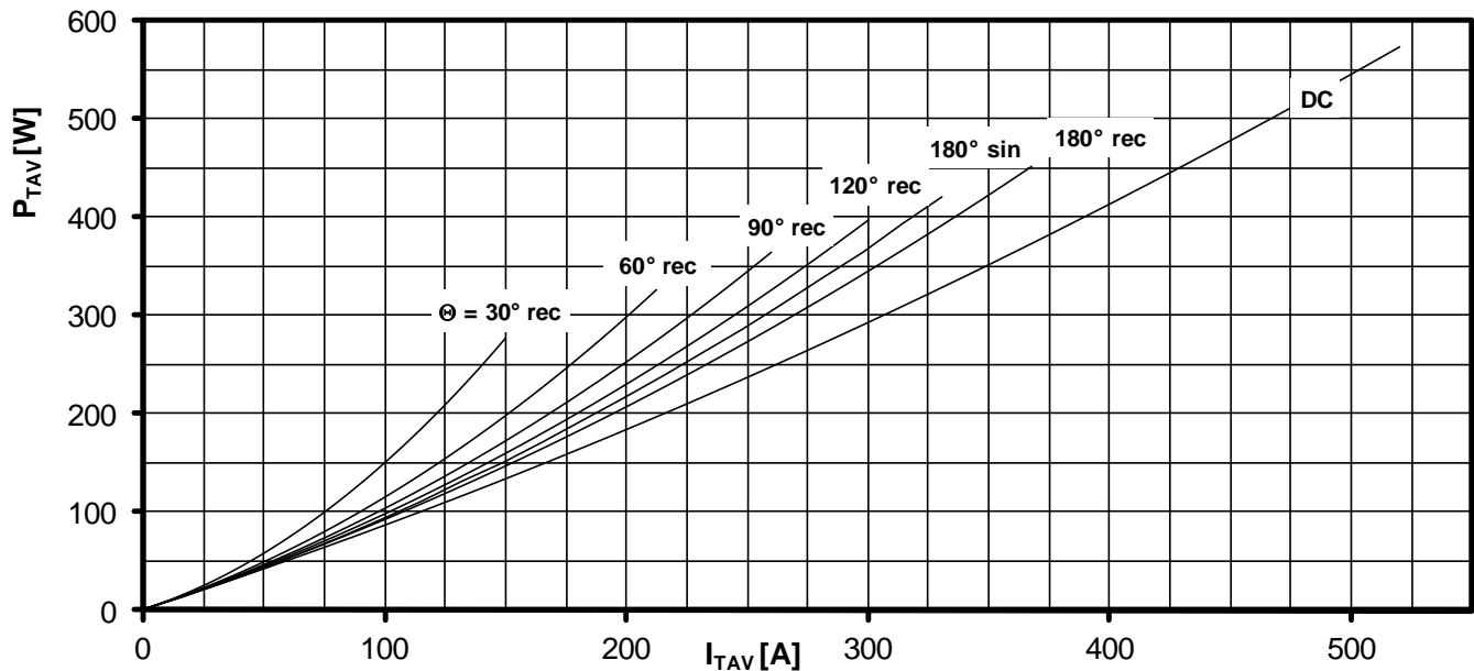
Durchlassverlustleistung je Zweig / On-state power loss per arm P_{TAV} = f(I_{TAV})
